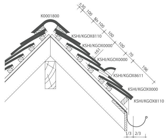
LENGTEDOORSNEDE DAK TER HOOGTE VAN VORST 1800 INGEMORTELD
