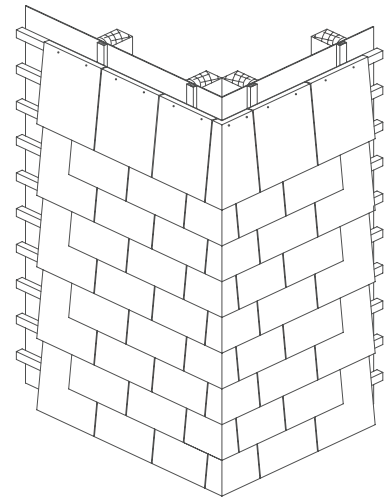
* 3D TEKENING GEVELBEKLEIDING MET DOORSNEDE
