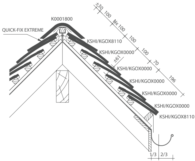
LENGTEDOORSNEDE DAK TER HOOGTE VAN VORST 1800 QUICK-FIX EXTREME
