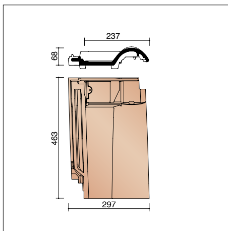
BROM8100 4,2 stuks/lm Ondervorstpan
