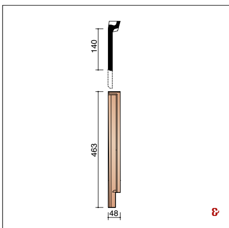
BROM7060 2,7 stuks/lm Individuele linker gevelplaat
