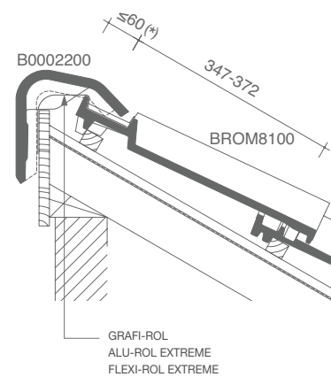
DWARSDOORSNEDE DAK TER HOOGTE VAN UNIVERSELE HAAKVORST
