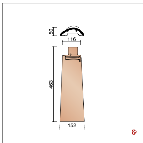
BROM8010 2,7 stuks/lm Halve pan
