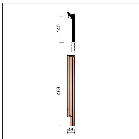
BROM7070 2,7 stuks/lm Individuele rechter gevelplaat
