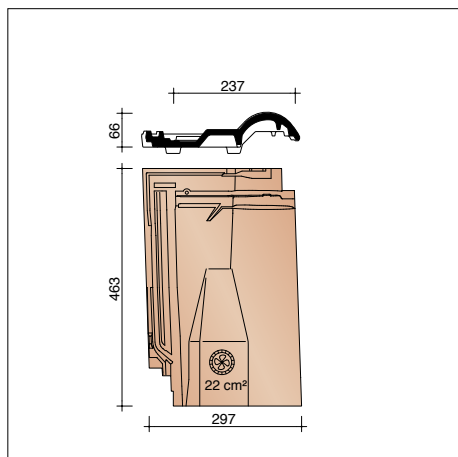
BROM8640 Ventilatiepan met rooster in kunststof 22 cm 2
