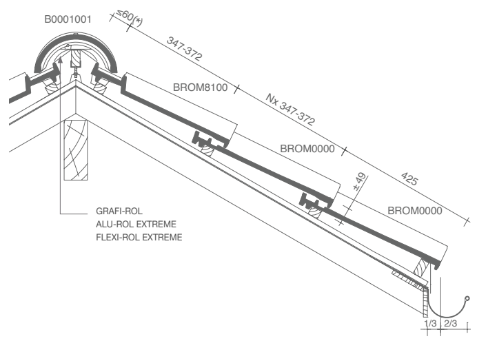
LENGTEDOORSNEDE DAK TER HOOGTE VAN VORST ONDERVORSTPAN
