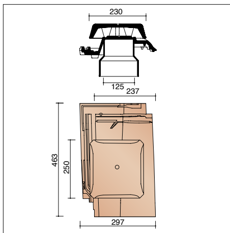
BROM8728 Kit kokerpan Ø 125 mm + kapje + aansluitingsmodule
