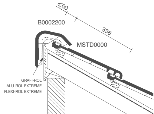
LENGTEDOORSNEDE DAK TER HOOGTE VAN UNIVERSELE HAAKVORST
